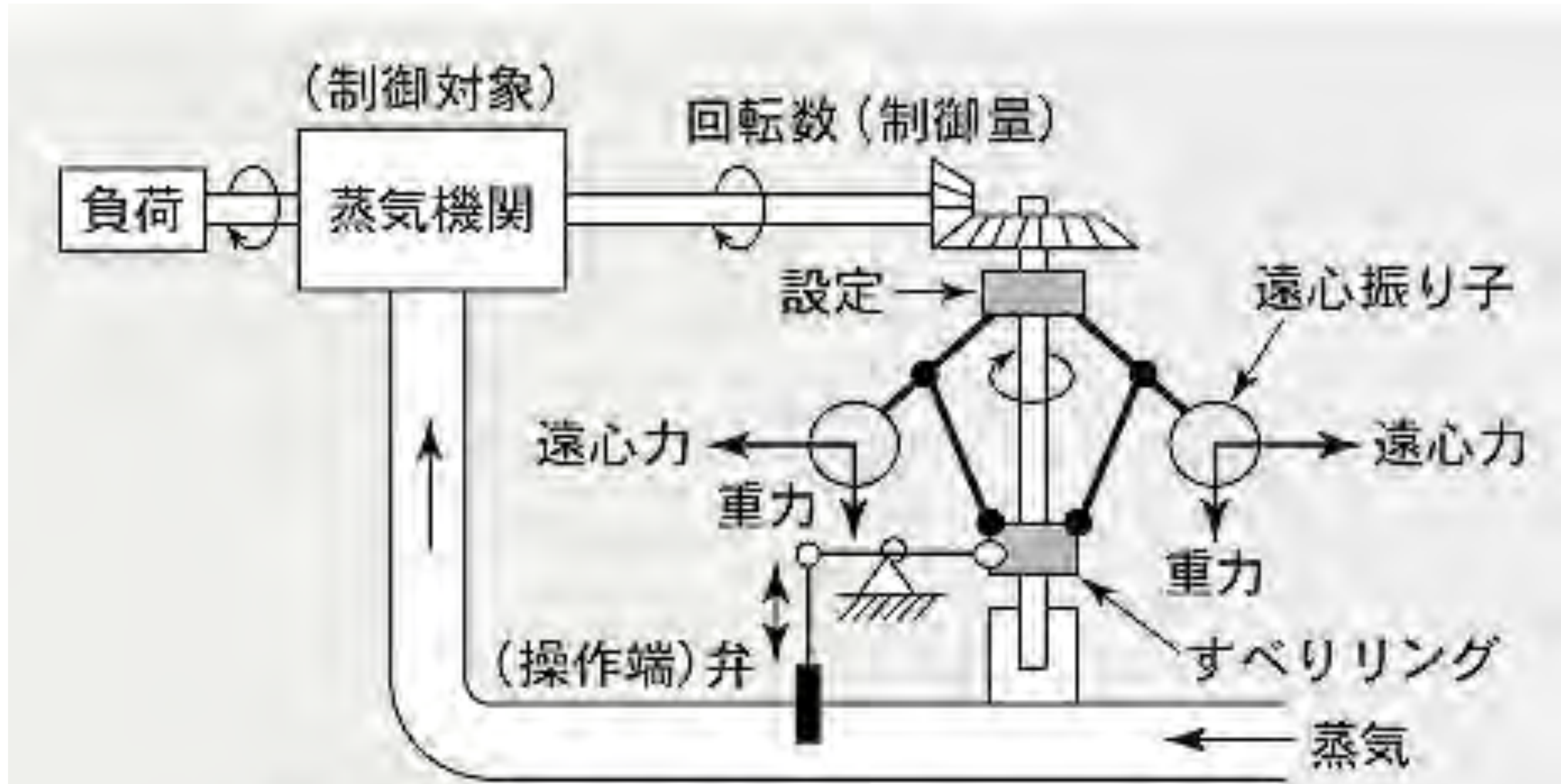
図1 蒸気機関の自動回転数制御の原理
